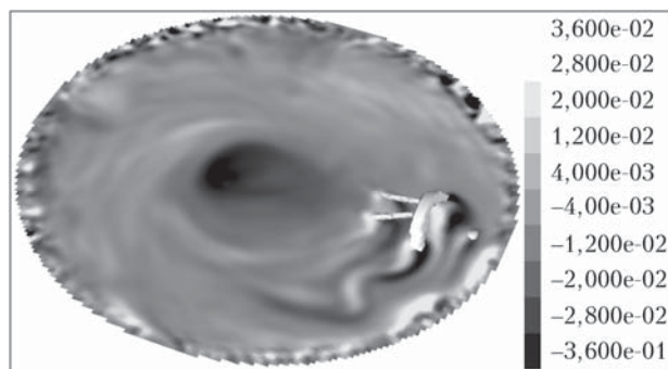
Рис. 12. Горизонтальное сечение поля вертикальной компоненты завихренности воздушной среды (rot\mathbf{U})_y , s^{-1} . Описание см. на рис. 11
