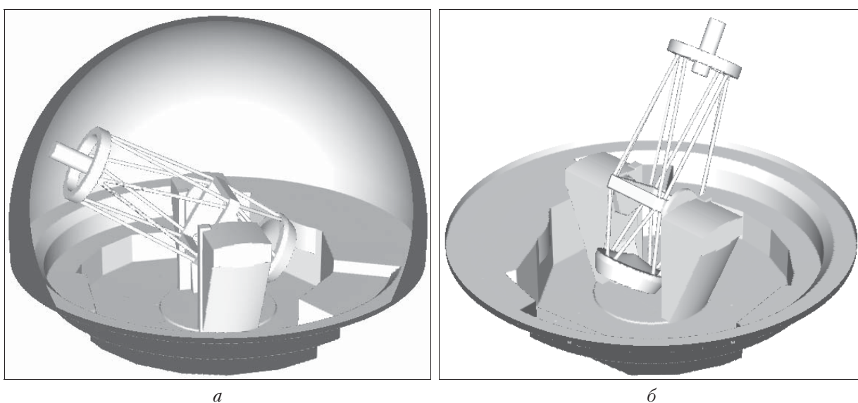
Рис. 9. Объемная масштабная модель помещения подкупольного пространства БТА, купол показан частично: а — азимутальный угол монтировки телескопа 270^\circ (на запад), зенитный угол трубы телескопа 60^\circ , вид с юга; б — азимутальный угол 225^\circ (на юго-запад), зенитный угол 30^\circ , вид с северо-запада
