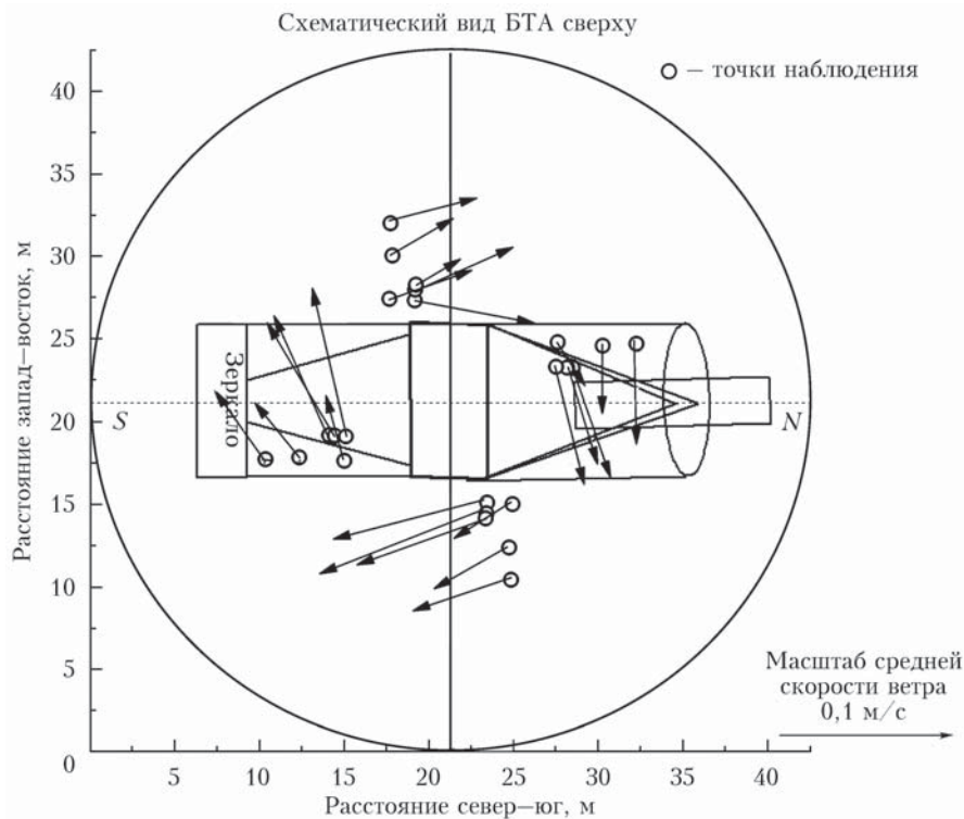
Рис. 6. Экспериментальное поле скоростей воздушных потоков в БТА на высотах 7\text{--}19 м при закрытом куполе 3.08.2016 г.
