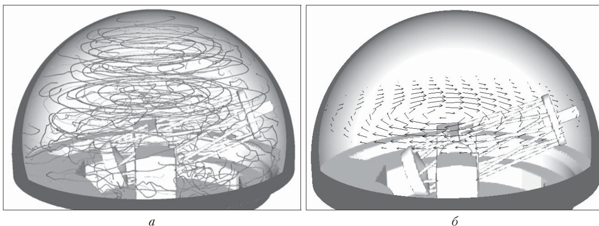
Рис. 10. Вихревая структура под куполом БТА. Момент времени моделирования 01:56:13. Азимутальный угол монтировки 270^\circ , зенитный угол трубы телескопа 70^\circ . Ближняя часть купола не показана, вид с севера: а — линии тока; б — горизонтальное сечение поля скоростей воздушных потоков на высоте 17 м
