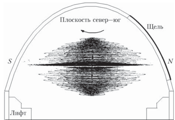
Рис. 5. Схематический вид вихревой структуры в подкупольном пространстве БТА, восстановленный из экспериментальных данных
