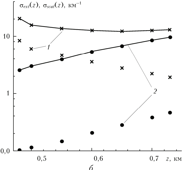
Рис. 2. Коэффициенты рассеяния (символы) и ослабления (линии с символами) излучения с длиной волны 41 мкм для модели 2: 1 – рассеивающий слой, состоящий из мелких и крупных капель; 2 – рассеивающий слой из мелких капель (а); аналогичные данные для излучения с длиной волны 200 мкм (б)
