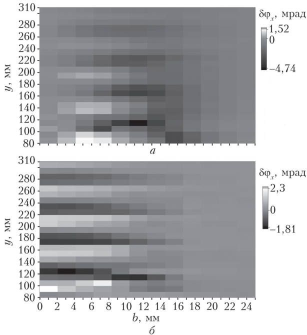
Рис. 4. Образы сверхзвуковой недорасширенной струи по данным лазерного просвечивания: a – горизонтальные, b – вертикальные отклонения
