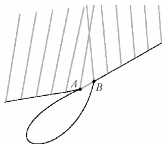
Рис. 3. Отклонение траектории движения рабочей точки от предполагаемого отрезка переезда. Здесь А – начало, а В – конец одного отрезка задания. Линии, направленные от точек задания вверх, – нормали к обрабатываемой поверхности
