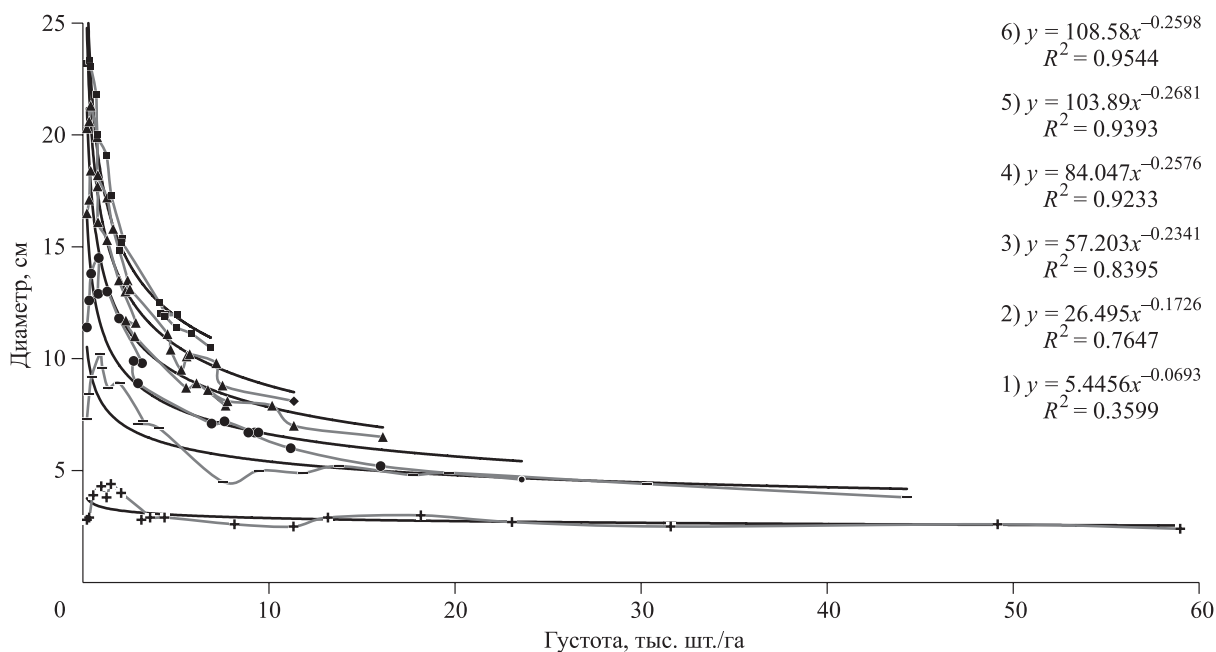
Рис. 2. Зависимость среднего диаметра лиственничных ценозов от их текущей густоты в возрасте, лет: 1 – 12; 2 – 17; 3 – 20; 4 – 25; 5 – 30; 6 – 35.
