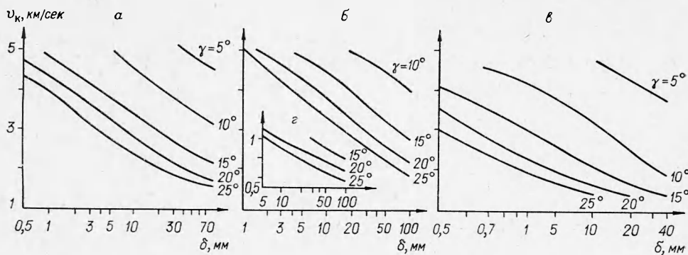
Рис. 4. Зависимость v_k^* от толщины свариваемых пластин при \delta_1/\delta_2=1 .
