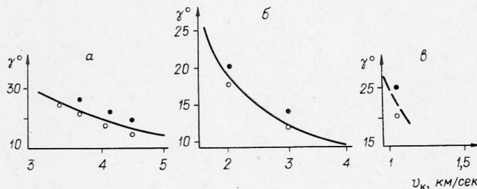
Рис. 5. Верхняя граница области сварки (расчет с k=0,37 ).
