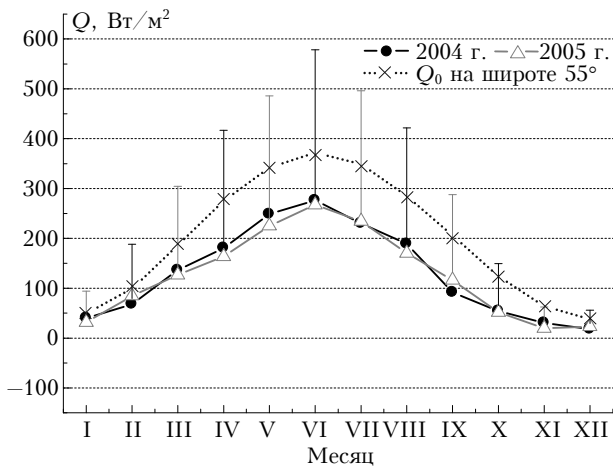
Рис. 2. Годовой ход суммарной солнечной радиации в г. Томске в 2004 и 2005 гг. и максимально возможная ее величина на широте 55°
