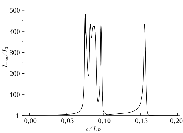
Рис. 5. Значение нормированной (на начальное значение) интенсивности светового поля на оси пучка R_0 = 2 \text{ мм} , P_0 = 10P_c , F = 0,1L_R вдоль дистанции распространения в рамках стационарной модели
