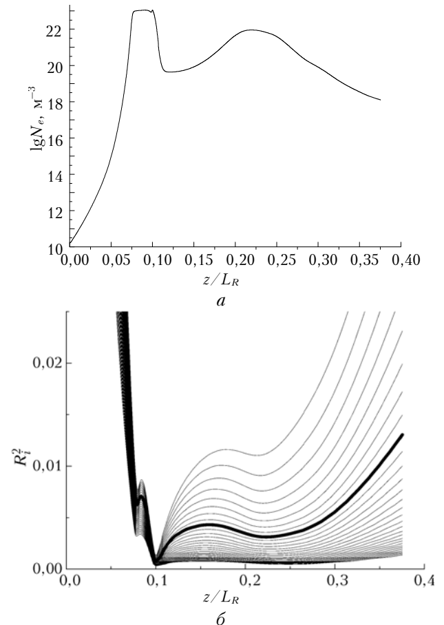
Рис. 4. Концентрация свободных электронов на оси лазерного пучка (а) и ход эффективных радиусов (нормированных на радиус всего пучка) дифракционно-лучевых трубок (б) вдоль дистанции распространения излучения с начальной пиковой мощностью 10P_c и радиусом R_0 = 1 мм. Жирной линией выделен эффективный радиус дифракционного луча, соответствующий границам поперечной дифракционно-лучевой трубки
