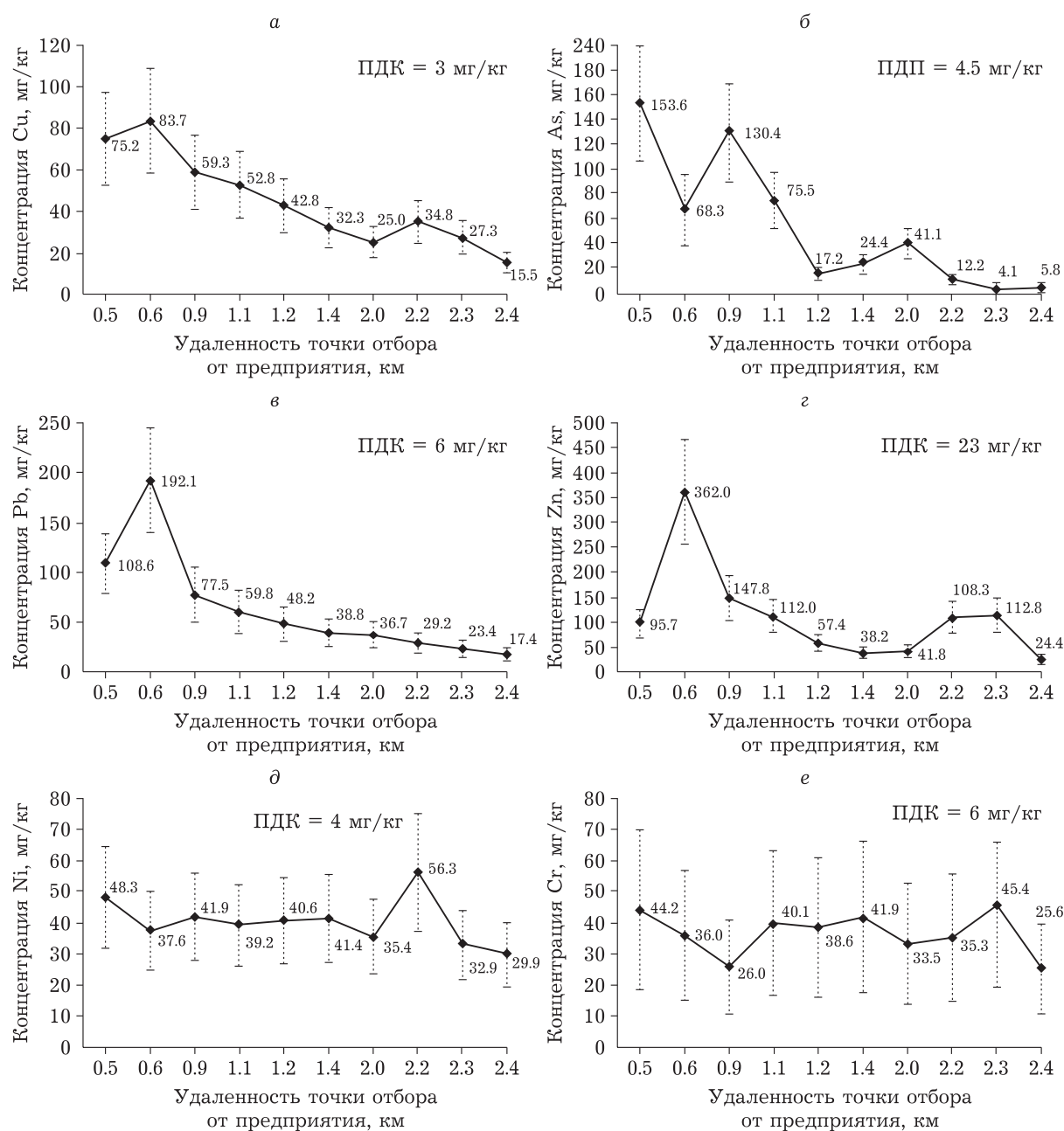
Рис. 2. Зависимость концентраций тяжелых металлов от удаленности точек отбора проб от Новосибирского оловянно-го комбината (количество почвенных образцов – 10, количество параллельных измерений – 3, P = 0.95 ).
