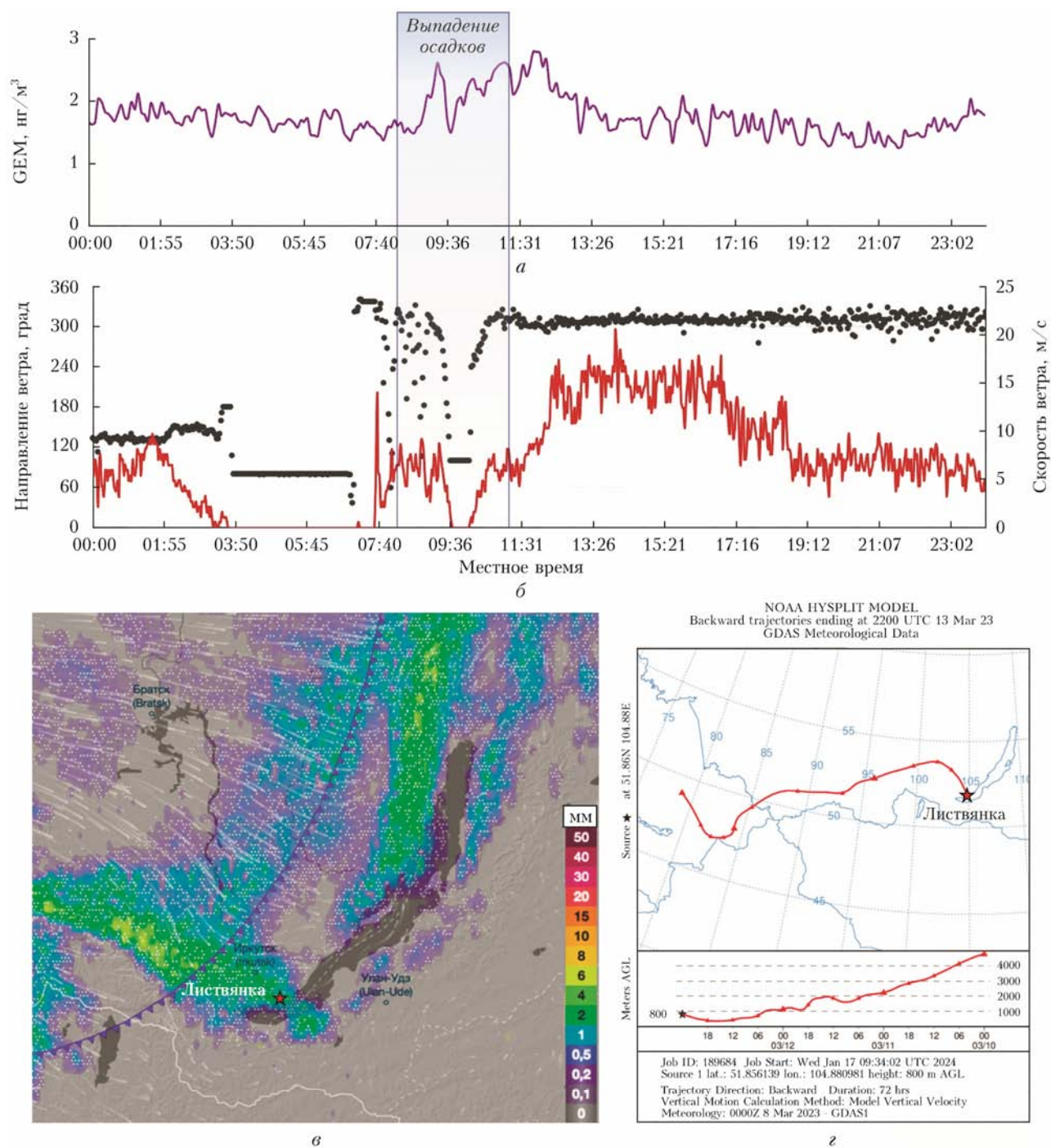
Рис. 6. Изменчивость GEM в атмосфере на ст. Листвянка 13.03.2023 г. (а); скорость и направление ветра в районе ст. Листвянка 13.03.2023 г. (б); карта осадков в 08:00 13.03.2023 г. ( https://www.ventusky.com ) (в); обратная траектория движения воздушных масс на высоте 800 м над уровнем земли в 08:00 13.03.2023 г. (цв. рисунки см. на сайте https://www.ready.noaa.gov/HYSPLIT.php ) (г)
