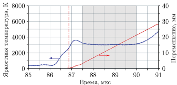
Зависимости яркостной температуры и перемещения детонационного фронта в ТНТ от времени
