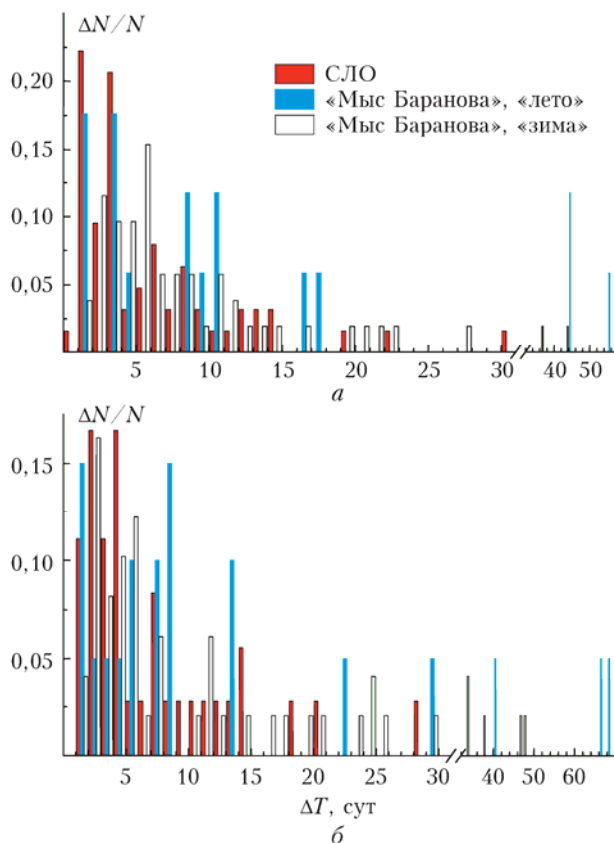
Рис. 3. Гистограммы распределений интервалов времени аномальных концентраций еВС (а) и V_f (б)
