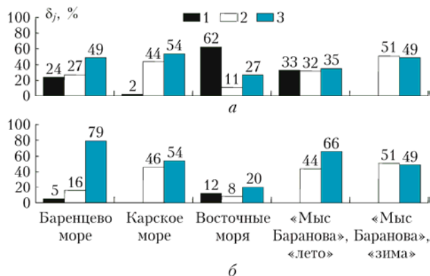
Рис. 4. Относительный вклад отдельных типов загрязнений в аномальные значения еВС (а) и V f (б) в четырех районах СЛО
