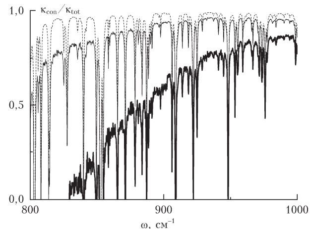
Рис. 7. Отношение непрерывного вклада к полному коэффициенту поглощения водяного пара в области окна 8–12 мкм. Пунктирная кривая — B_{\text{con}} = 500 \text{см}^{-1} , тонкая кривая — 600 \text{см}^{-1} ; полужирная кривая — 700 \text{см}^{-1}
