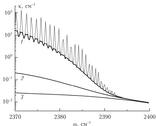
Рис. 4. Коэффициент поглощения в крыле полосы 4,3 мкм CO_2 , T = 296 К, P_{CO_2} = 1 атм. Тонкая кривая — полный коэффициент, рассчитанный с контуром АТКЛ, полужирные кривые — коэффициент континуального поглощения, полученный вычитанием локального вклада линий с контуром АТКЛ: 1 — B_{con} = 0,3 ; 2 — 10; 3 — 25 cm^{-1} . Шаг по частоте 0,2 cm^{-1}
