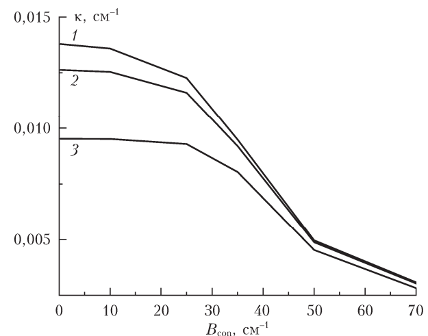
Рис. 8. Коэффициент непрерывного поглощения \text{CO}_2 при самоуширении для нескольких частот в крыле полосы 4,3 мкм при изменении границы локального вклада линий: 1 — 2395; 2 — 2396; 3 — 2400 \text{см}^{-1}
