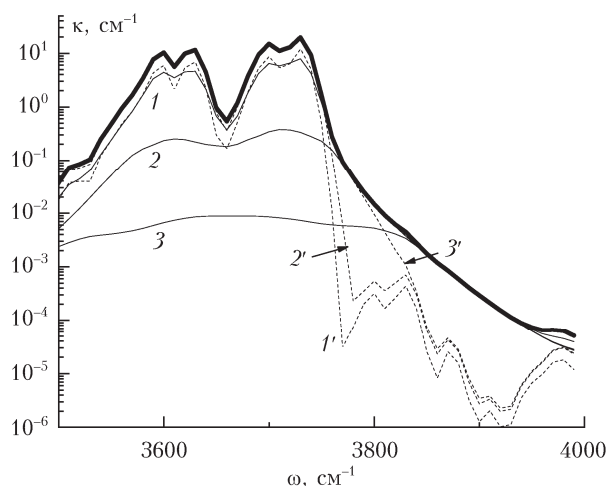
Рис. 5. Поглощение в области полосы 2,7 мкм CO_2 . Полушириная кривая — полный коэффициент поглощения; кривые 1–3 — континуальное поглощение при B_{con} = 5, 25, 100 cm^{-1} ; кривые 1'–3' — локальный вклад линий в поглощение при B_{con} = 5, 25, 100 cm^{-1} ; P_{CO_2} = 21,685 атм
