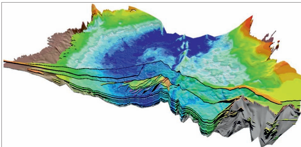
Рис. 3. Цифровой структурный каркас центральной части Западной Сибири.
