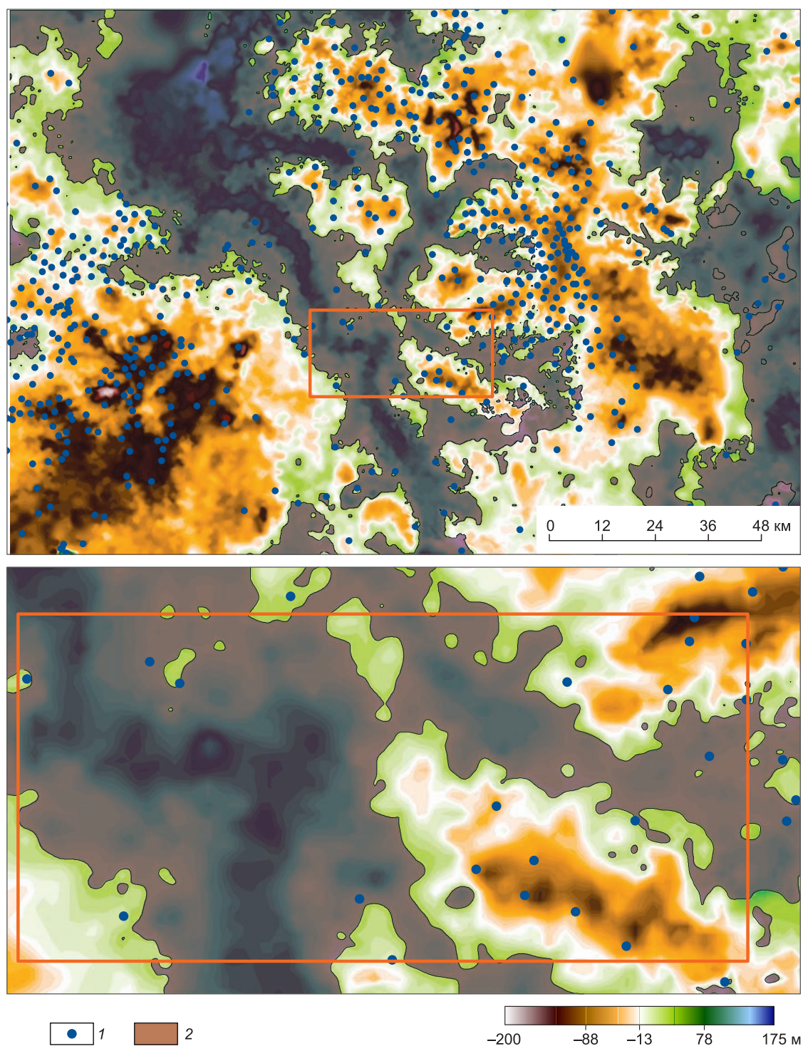
Рис. 2. Нижнеюрские отложения в районе Красноленинского свода.
