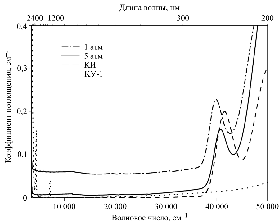
Рис. 1. Спектры поглощения кварцевых стекол, полученных из крупки кристобалита «суперкварцита», проплавленных при давлении 1 и 5 атм, в сравнении с поглощением стекол марки КИ и КУ-1.
