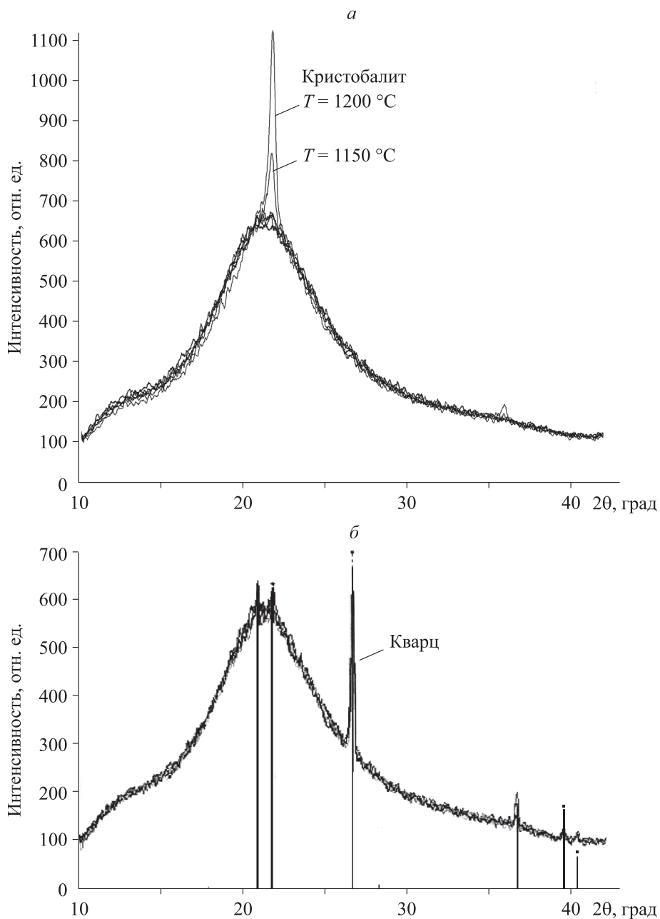
Рис. 2. Спектры рентгенофазового анализа кварцевого стекла, полученного из крупки «суперкварцита», в процессе термических испытаний (а) и истертого кварцевого стекла, отожженного при температуре T = 1200\text{ }^{\circ}\text{C} в течение 2 ч (б).
