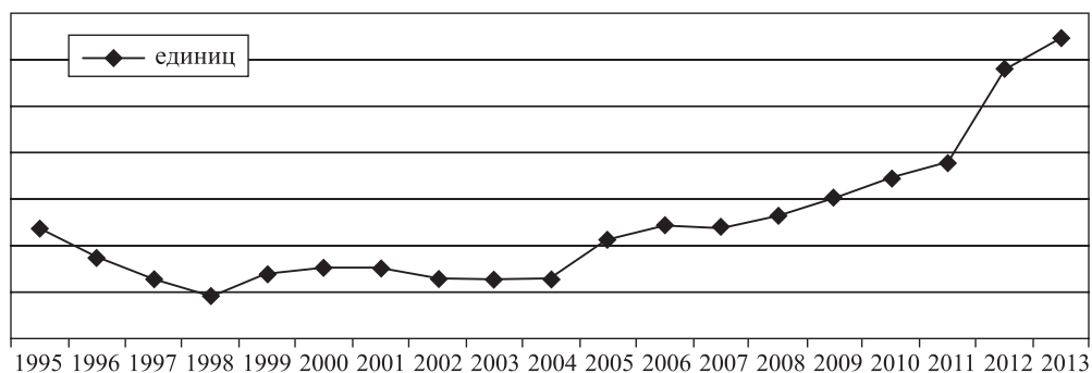
Рис. 1. Число субъектов малого предпринимательства в Республике Хакасия за 1995–2013 гг.
