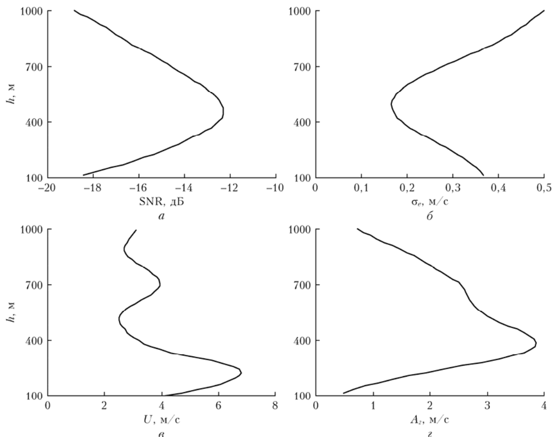
Рис. 2. Высотные профили SNR ( а ), инструментальной погрешности оценки вертикальной составляющей вектора скорости ветра ( б ), горизонтальной составляющей вектора скорости ветра ( в ) и начальной амплитуды квазигармонических колебаний вертикальной составляющей вектора скорости ветра ( г ), восстановленные из измерений лидаром Stream Line в томском Академгородке с 19:44 до 20:14 по местному времени 07.07.2023 г. при прохождении БГВ
