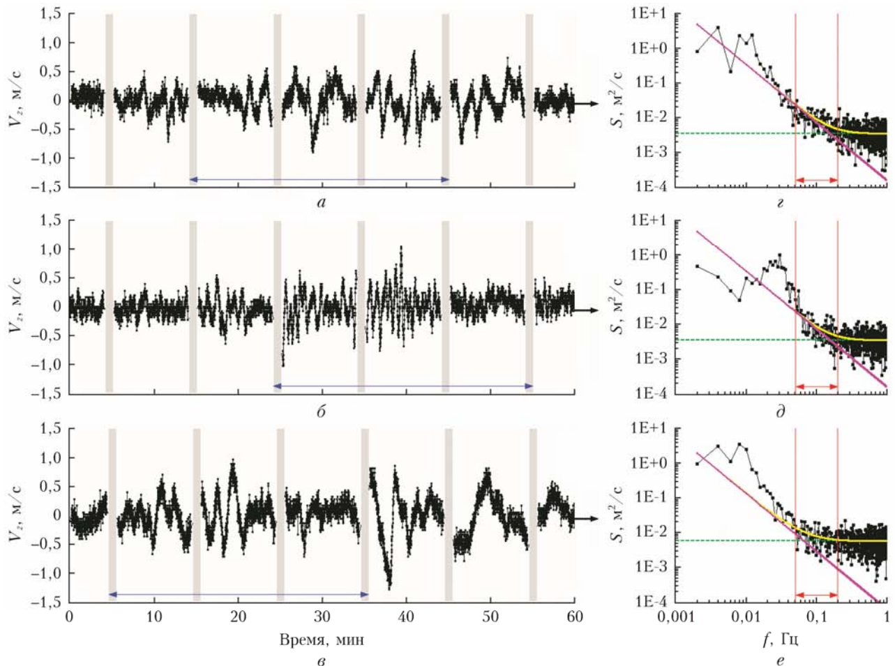
Рис. 5. Часовые вариации вертикальной компоненты вектора скорости ветра на высоте 350 м, полученные из измерений лидаром Stream Line в томском Академгородке с 06:00 ( а ), 07:30 ( б ) и 23:00 ( в ) по местному времени 06.10.2023 г., и рассчитанные по ним спектральные плотности V_z (черные кривые) в пределах временных интервалов, показанных синими стрелками ( з–е ): зеленые пунктирные линии указывают на шумовые составляющие спектров; красными стрелками показан частотный интервал, в пределах которого из спектральных плотностей определялась \epsilon , по ней рассчитывались спектральные плотности с учетом шума и усреднения по зондируемому объему (желтые кривые) и « -5/3 -я» колмогоровская зависимость спектра от частоты (розовые линии)
