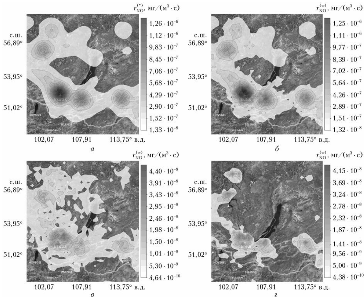
Рис. 1. Сравнение «истинного» распределения источников r_{\text{NO}}^{(*)} (а) и результатов его оценки алгоритмом усвоения данных r_{\text{NO}}^{(\infty)} в окне усвоения [16 \times 3600, 24 \times 3600] с ограничением на расположение источника (б) и без него (в), а также результатов решения обратной задачи (г) без ограничения для \theta_{\text{Snapshot}}^{(x)} \times \theta_{\text{Snapshot}}^{(y)} = 22 \times 22
