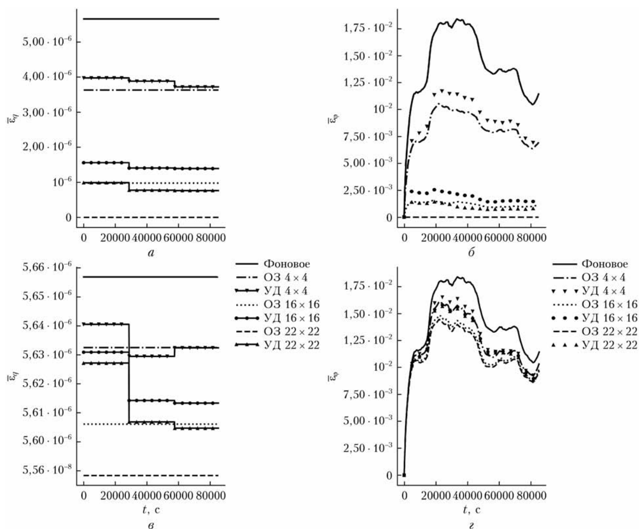
Рис. 3. Зависимость от модельного времени абсолютной ошибки восстановления источников NO ( r_{NO} ) (а, в) и динамики полей концентраций ( \varphi_{NO} ) (б, г) алгоритмом усвоения данных с окном усвоения 8 ч и решения обратной задачи для различных значений \theta_{Snapshot}^{(x)} \times \theta_{Snapshot}^{(y)} с ограничением по вертикали (а, б) и без него (в, г); сплошная линия (Фоновое) соответствует решению без использования методов обратного моделирования \varphi[q^{(0)}] (с нулевым источником)
