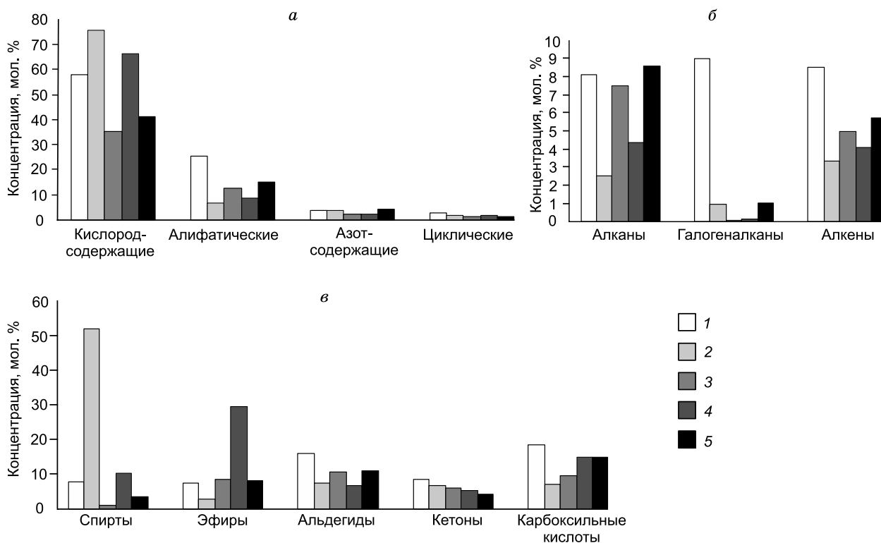
Рис. 4. Относительные содержания углеводородов во вкрапленниках плагиоклаза (1) и оливина (2) из базальтов, кварца (3), клинопироксена (4) и ортопироксена (5) из риолитов влк. Меньший Брат:
