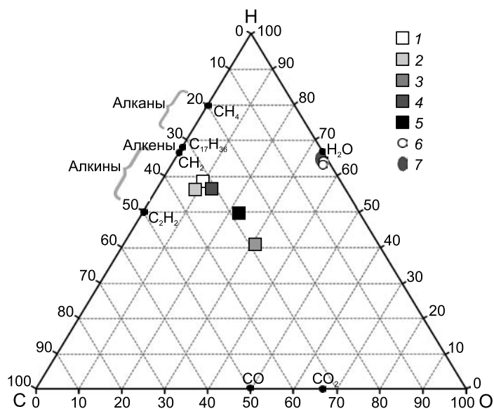
во вкрапленниках плагиоклаза (1) и оливина (2) из базальтов, кварца (3), клинопироксена (4) и ортопироксена (5) из риолитов влк. Меньший Брат на диаграмме С—О—Н в сравнении с составами фумарольных газов активных вулканов Горелый (Камчатка) (6) и Кудрявый (кальдера Медвежья, о. Итуруп) (7).
