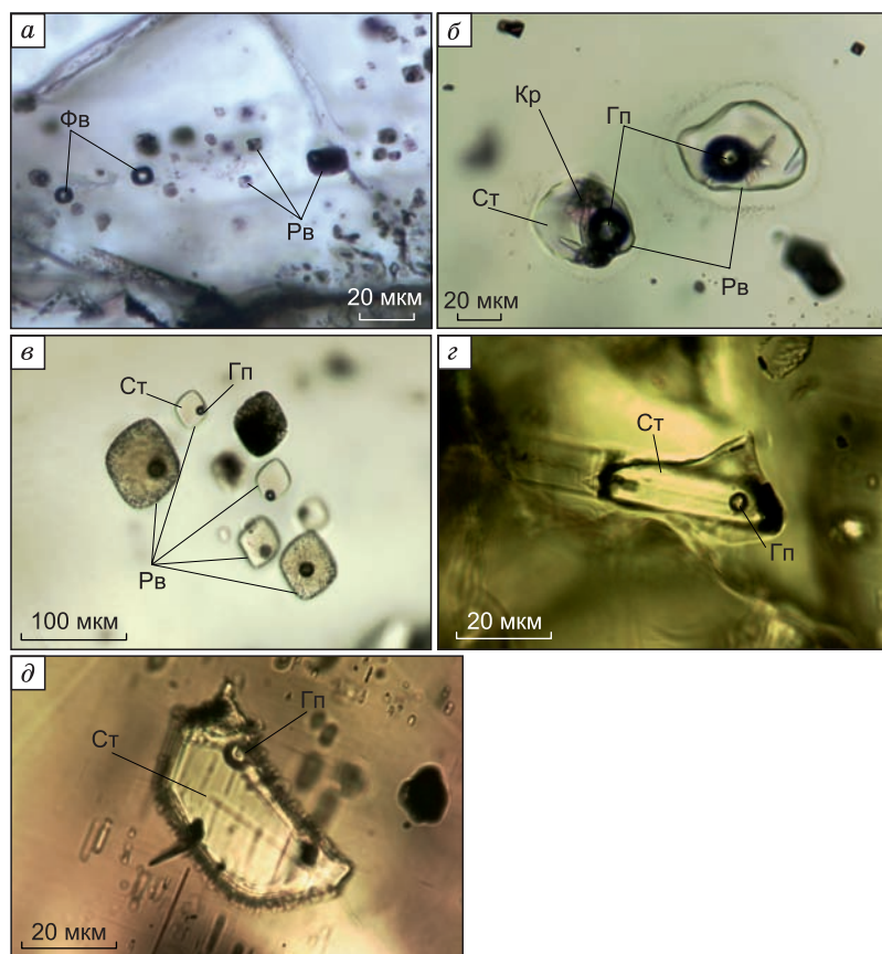
Рис. 2. Фото включений минералообразующих сред во вкрапленниках базальтов влк. Меньший Брат:
