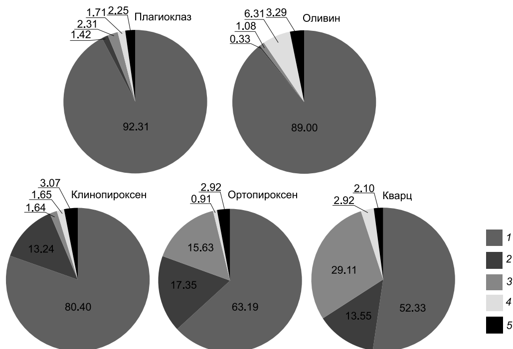
Рис. 3. Содержания (мол. %) летучих компонентов газовой фазы флюидных и расплавных включений во вкрапленниках базальтов и риолитов влк. Меньший Брат, о. Итуруп:
