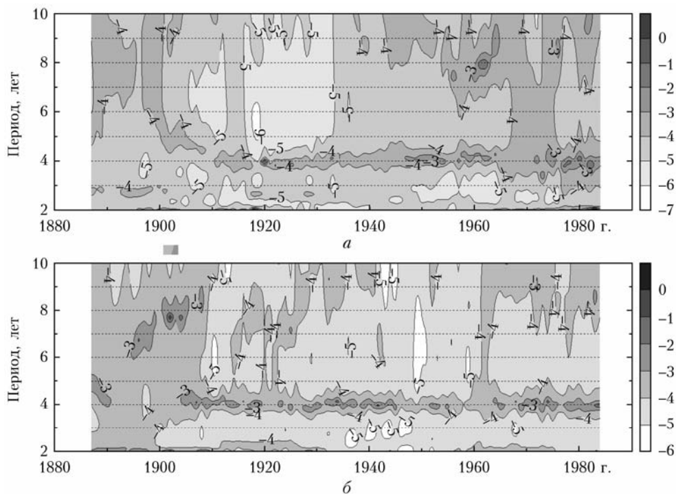
Рис. 4. Скользящий спектр содержания \text{CO}_2 (а) и \text{H}_2\text{O} (б) в годовых кольцах кедра у д. Трубачево (10 км к юго-востоку от г. Томска). Единицами цветовой шкалы являются десятичные логарифмы спектральной плотности температур ( ^{\circ}\text{C}^2/\text{год} ) (а) и осадков ( \text{мм}^2/\text{год} ) (б)
