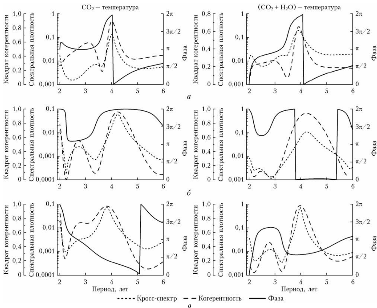
Рис. 3. Кросс-спектры хронологий \text{CO}_2 и \text{CO}_2 + \text{H}_2\text{O} с температурой (за вегетационный период) для спилов лиственных деревьев: а – береза; б – черемуха; в – ива; г – липа; д – осина (окончание см. на с. 5)
