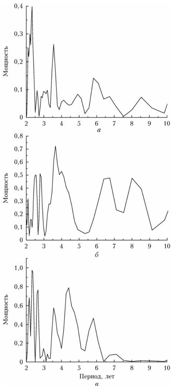
Рис. 1. Результат спектрального анализа индекса САК (1951–2023 гг.), осредненного: за 12 месяцев (а); за 4 зимних месяца (с декабря прошлого года по март текущего) (б); за вегетационный период (с мая по сентябрь текущего года) (в)
