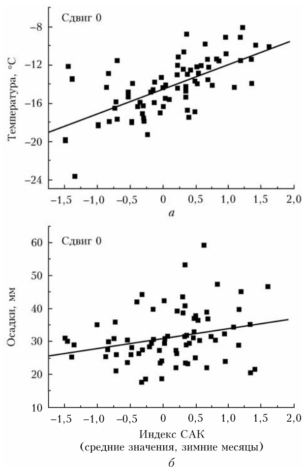
Рис. 2. Корреляционные диаграммы средних по четырем зимним месяцам температур (а) и сумм осадков (б) в г. Томске с индексом САК
