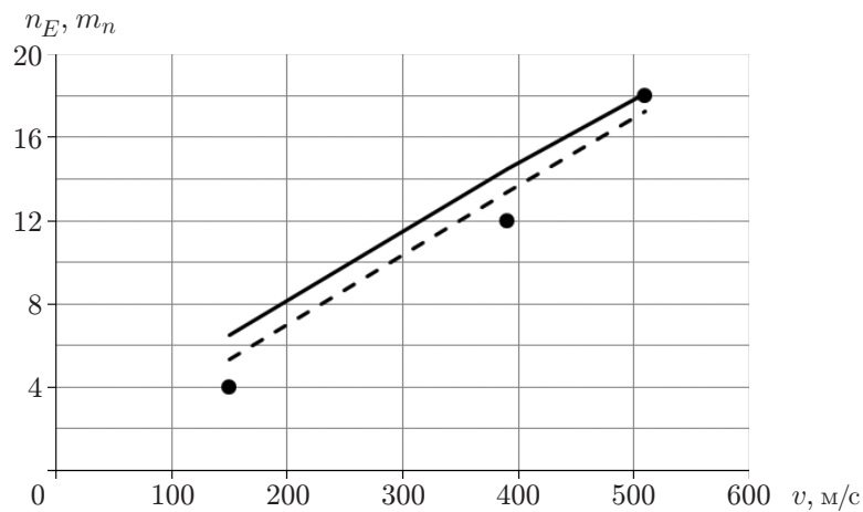
Рис. 4. Зависимость числа продольных разрывов от скорости расширения для оболочек из стали с массовой долей углерода 0,07 %:
