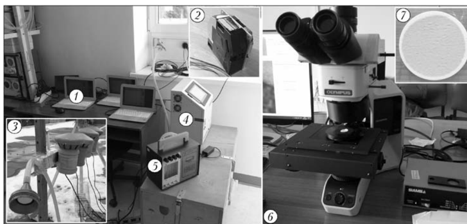
Рис. 1. Измерительно-исследовательский комплекс для анализа концентрации и фракционного состава атмосферного аэрозоля: ПК для регистрации данных (1); аэрозольный сенсор Panasonic PM 2.5 (2, 3); спектрометр ДАС 2702-М (4); аспиратор ПА-300М-2 (5); анализатор структуры твердых тел на основе оптического микроскопа Olympus BX-53 (6); фильтр Whatman EPM 2000 с отобранной пробой атмосферного аэрозоля (7)
