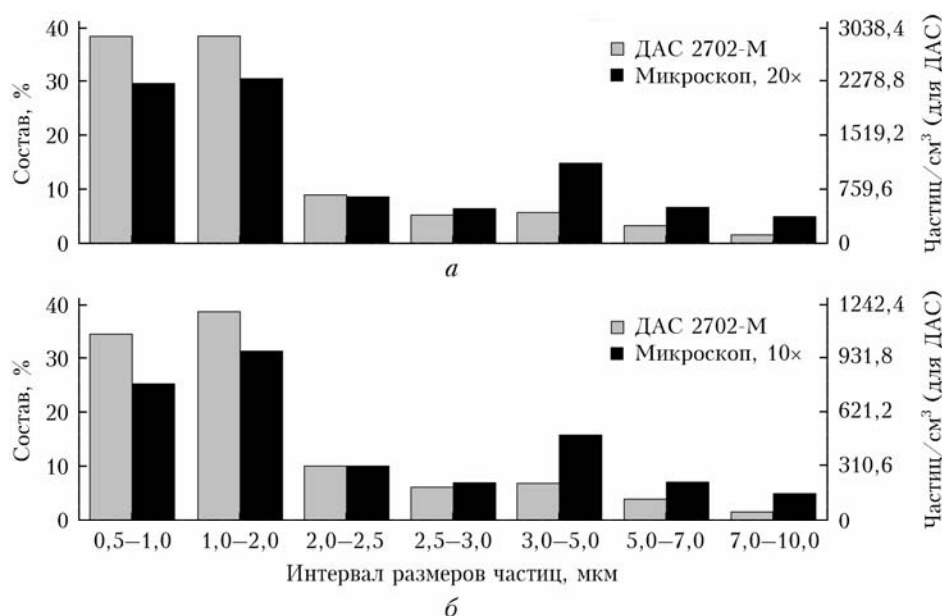
Рис. 4. Сравнение фракционного состава аэрозольных частиц по данным спектрометра и микроскопа: а – серия измерений № 1; б – серия измерений № 2
