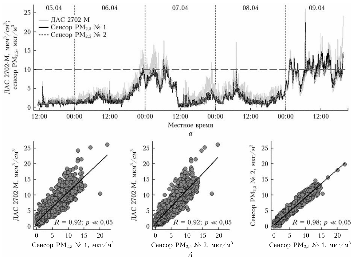
Рис. 3. Временные ряды (а) и диаграммы рассеяния (б) концентрации PM_{2.5} , измеренной с помощью сенсоров и ДАС 2702-М в приземной атмосфере Екатеринбурга с 5 по 9.04.2022 г. ( p – уровень значимости)
