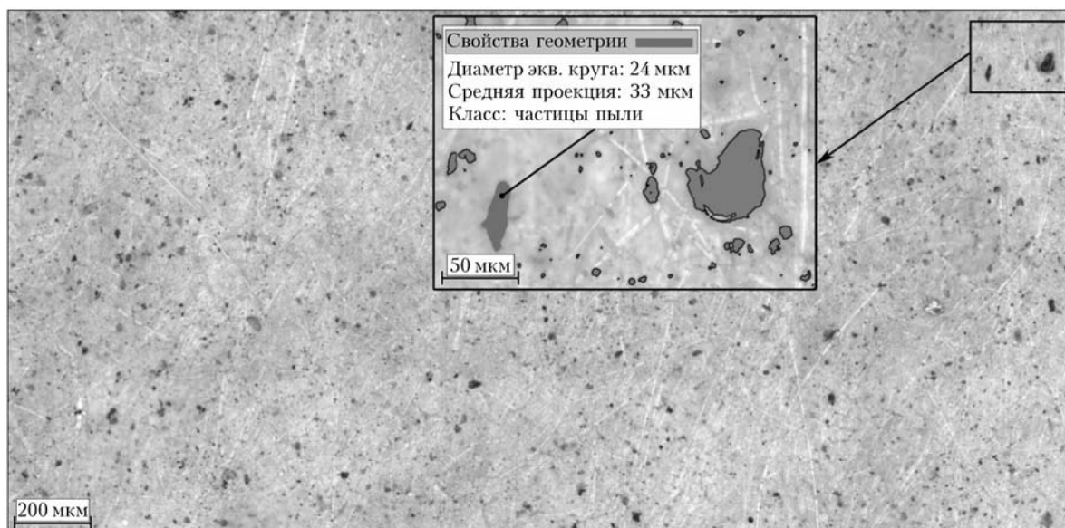
Рис. 2. Панорама участка поверхности фильтра, полученная с помощью микроскопа (на вставке — фрагмент с наложенными сегментационными масками)
