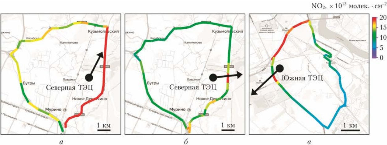
Рис. 1. Схемы маршрутов мобильных DOAS-измерений вокруг Северной и Южной ТЭЦ Санкт-Петербурга, проведенных 28.03.2016 г. (а), 16.03.2017 г. (б) и 19.04.2023 г. (в). Черными стрелками показано среднее направление ветра на высоте 150 м (см. табл. 1) (см. цветные рисунки на сайте http://iao.ru/ru/content/vol.37-2024/iss.10 )
