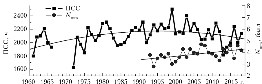
Рис. 1. Многолетние изменения балла нижней облачности и годовых значений ПСС
