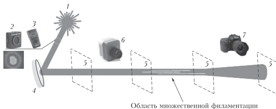
Рис. 1. Схема эксперимента: 1 — титан-сапфировый лазерный комплекс; 2 — измеритель профиля пучка LBP2-HR-VIS; 3 — измеритель энергии импульса ОРНІR-II; 4 — поворотное зеркало; 5 — экран; 6 — CCD-камера «ANDOR-Clara E»; 7 — фотокамера Pentax K-3
