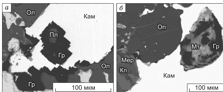
Рис. 5. Два типа выделений графита.
