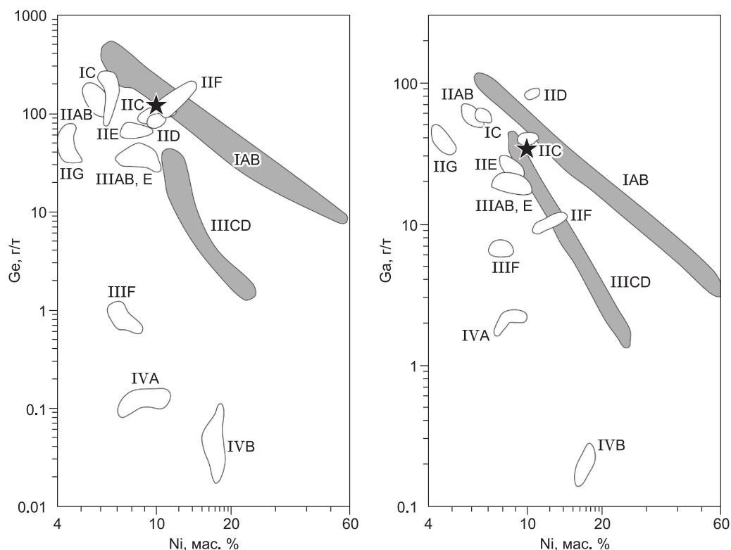
Рис. 8. Соотношение Ni, Ga и Ge в различных группах железных метеоритов, по данным работы [Goldstein et al., 2009].
