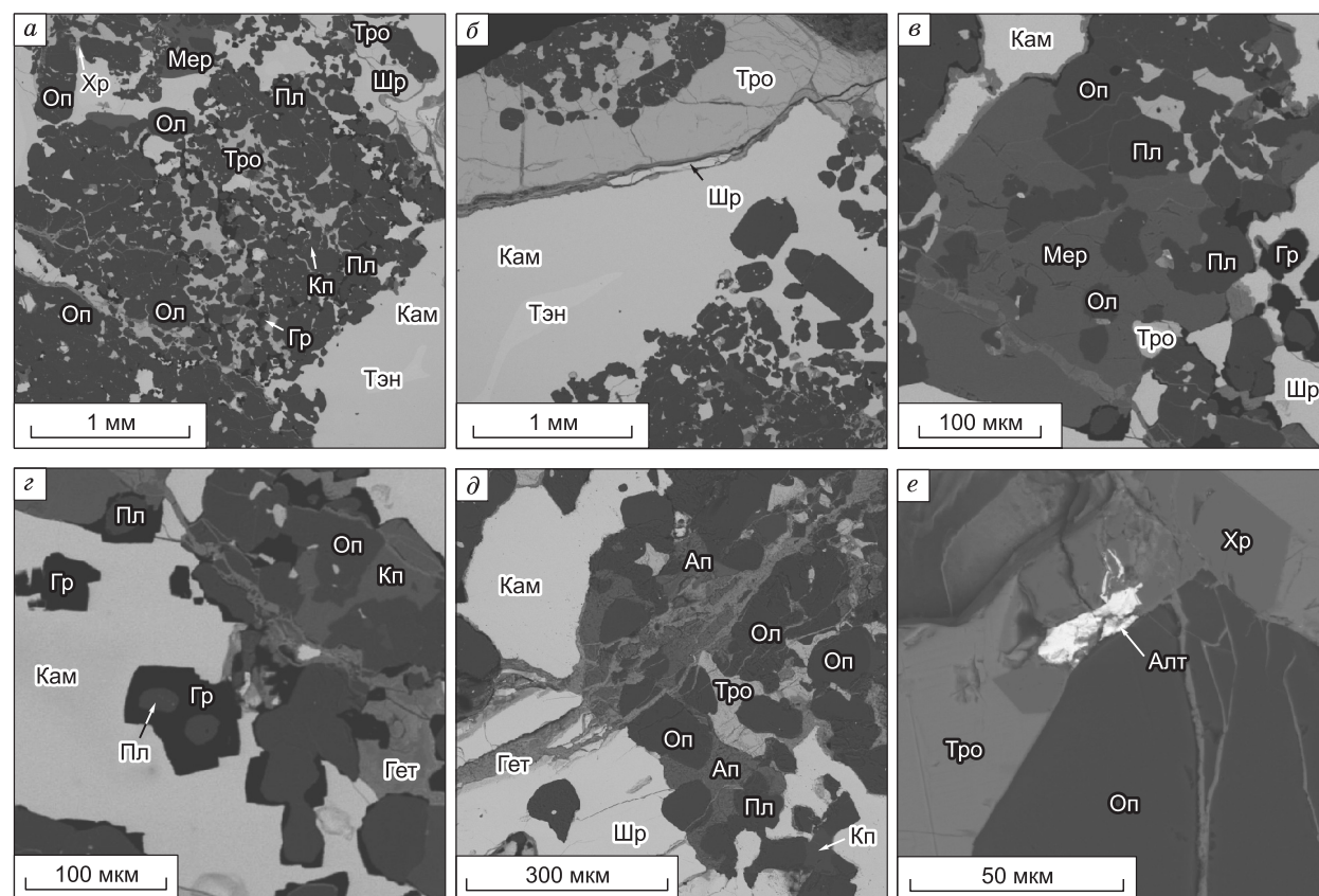
Рис. 3. Микроструктура силикатных включений:
