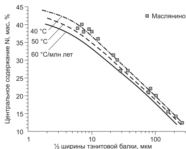
Рис. 12. Оценка скоростей остывания метеорита Маслянино по соотношению толщины балок тэнита и содержания Ni в центральной части.
