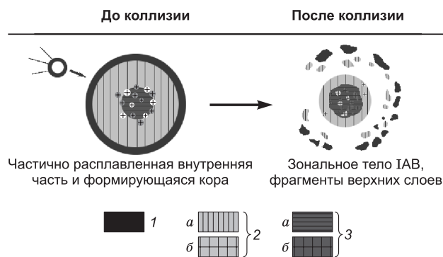
Рис. 13. Модель формирования метеоритов группы IAB (+HCD) и винонаитов в результате ударного распада и ре-аккреции родительского тела, по данным работы [Ruzicka, 2014] с изменениями.
