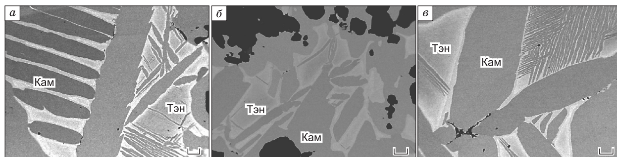
Рис. 2. Видманштеттенова структура выделений камасита (Кам) и тэнита (Тэн) в обр. Mas-4.
