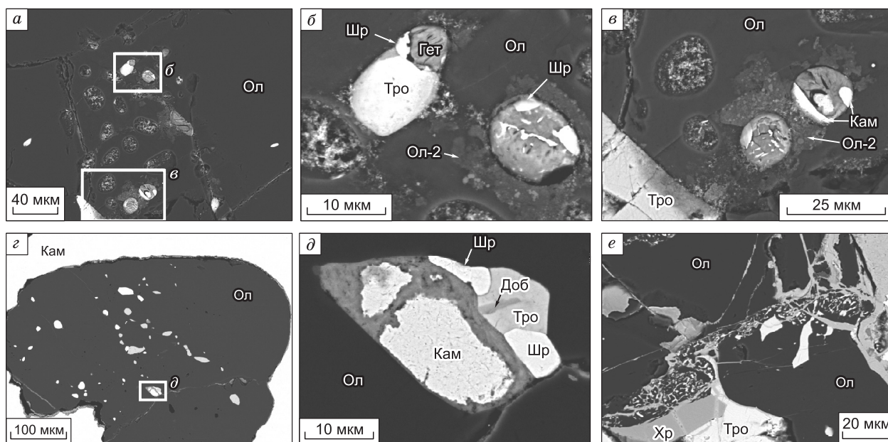
Рис. 4. a—d — зоны округлых включений в оливине обр. Mas-1; e — эмульсионная смесь троилита и хромита с оливином, обр. Mas-4.
