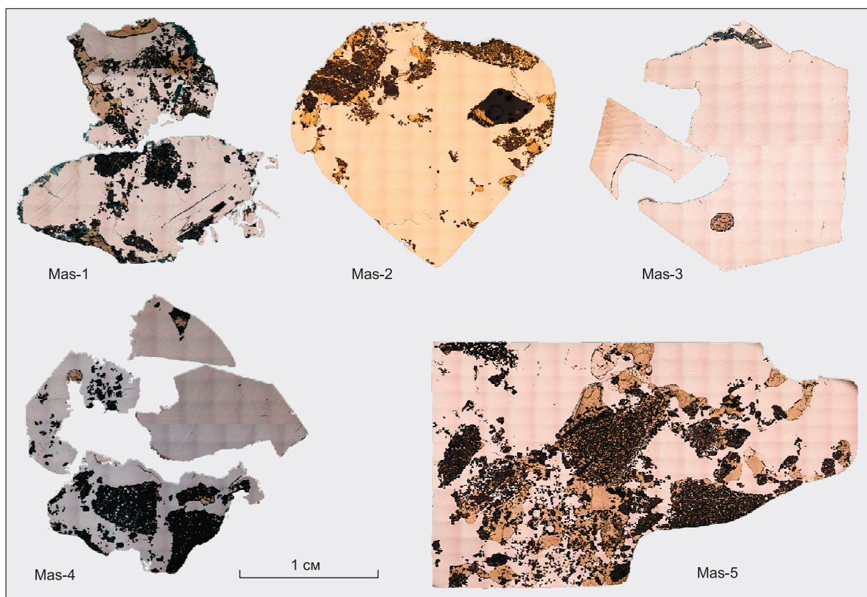
Рис. 1. Микрофотографии исследованных фрагментов метеорита Маслянино.
