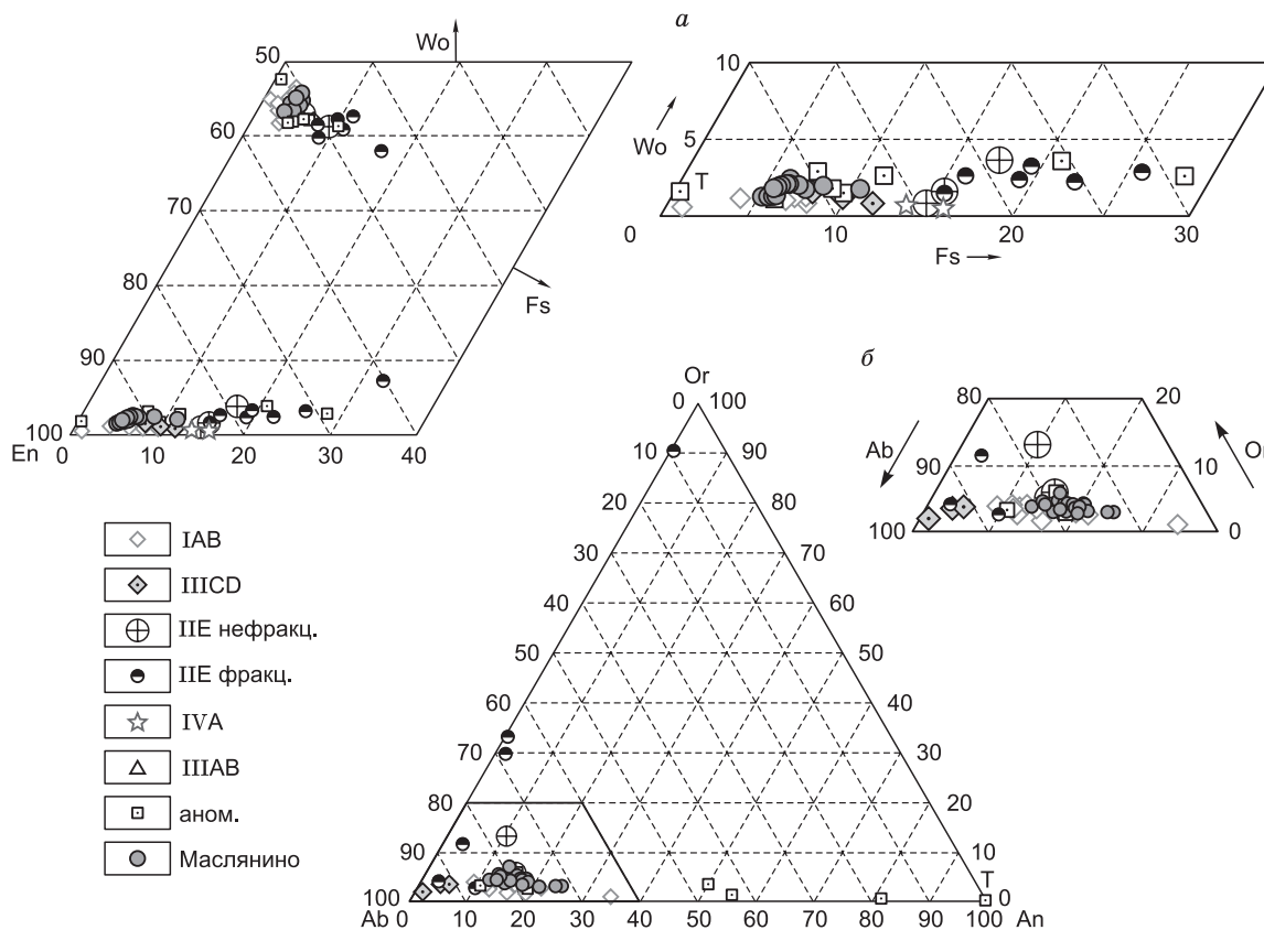
Рис. 7. Состав пироксенов ( a ) и плагиоклазов ( б ) в метеорите Маслянино в сравнении с другими группами железных метеоритов, по данным работы [Ruzicka, 2014].
