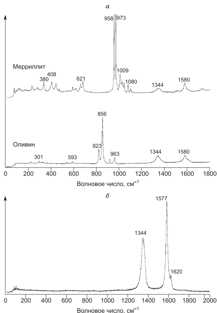
Рис. 11. Рамановские спектры оливина и мерриллита (а) и графита (б) из метеорита Маслянино.
