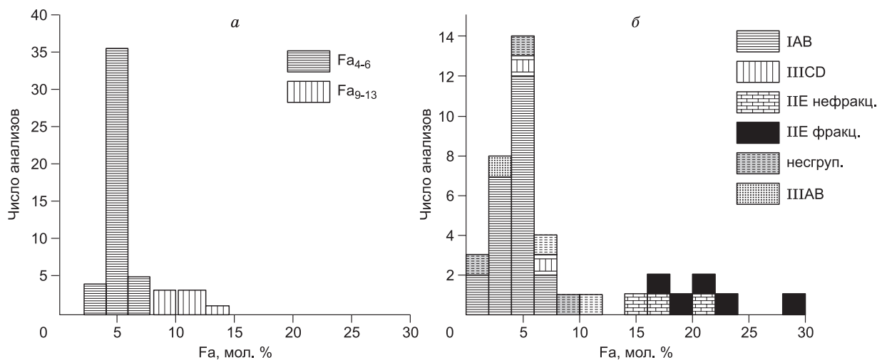
Рис. 6. Гистограммы распределения фаялитового минала в оливине в различных железных метеоритах:
