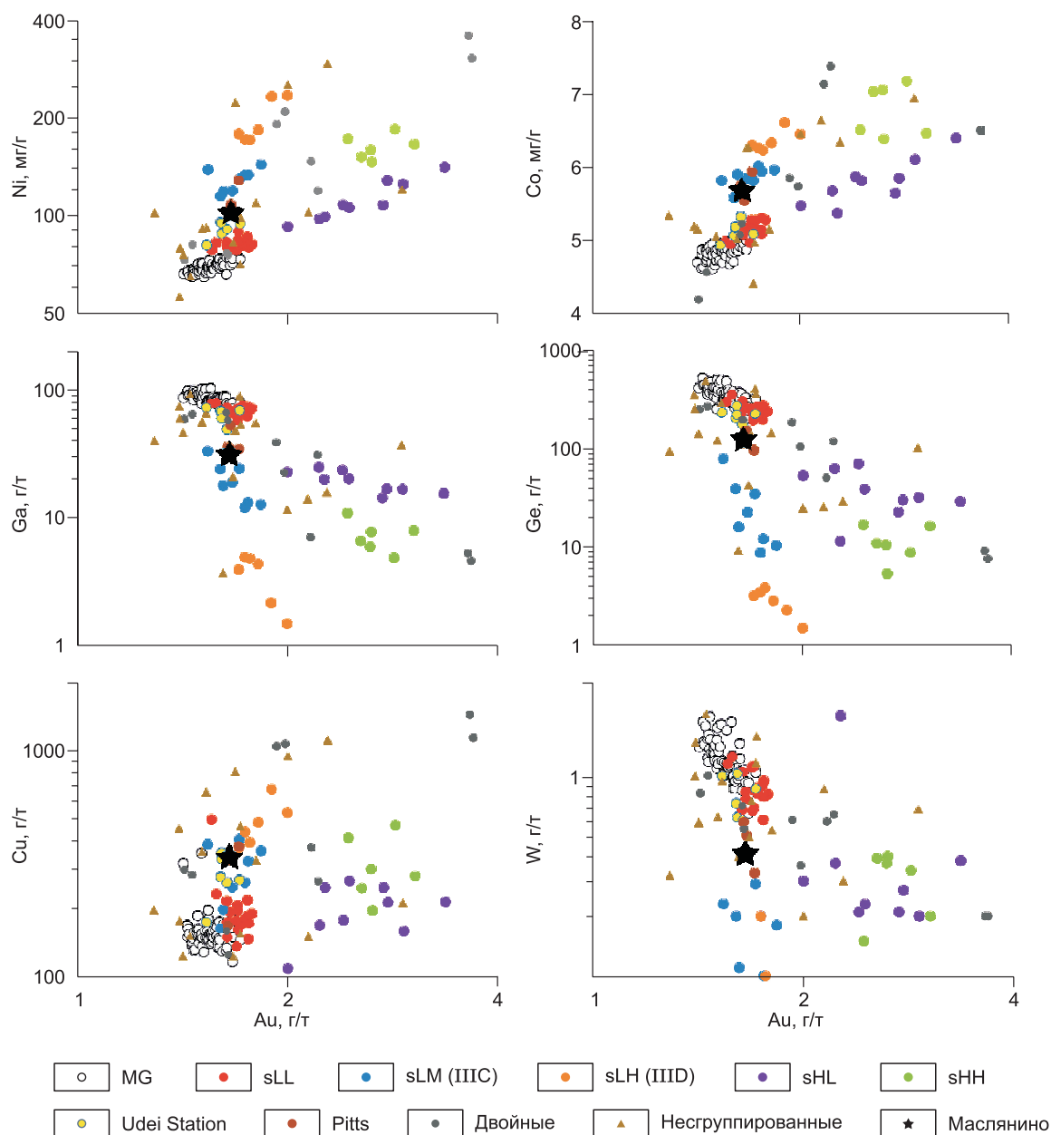
Рис. 9. Соотношение Au и других элементов в метеоритах группы IAB.
